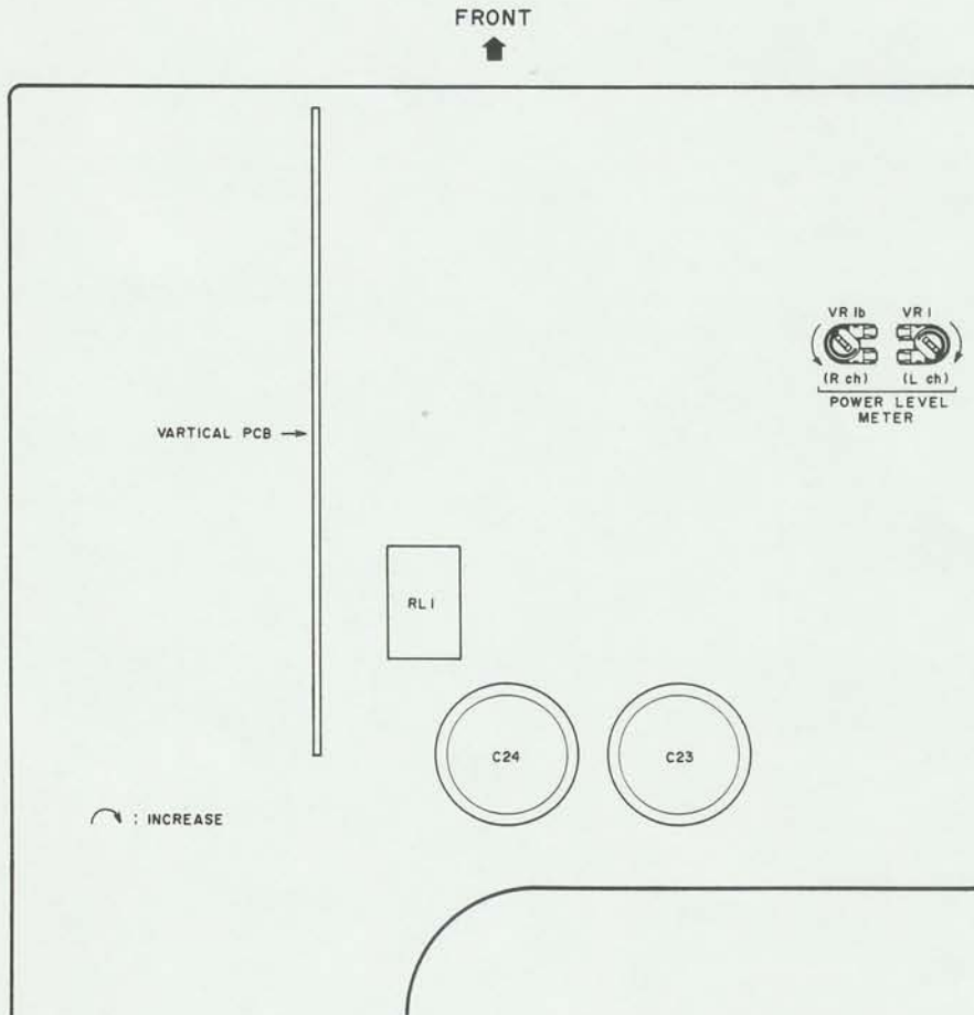
Fig. 6-2 Main-Amp PCB
