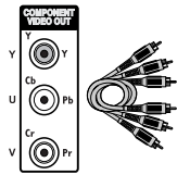
RCA-Buchsen und Kabel für Videosignal Y, Pb/Cb, Pr/Cr, auch Komponenten-Buchse/Kabel genannt.
